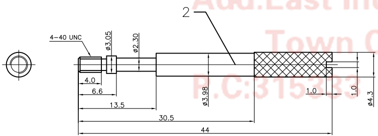
Long BOLT
