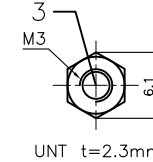
UNT t=2.3mm
