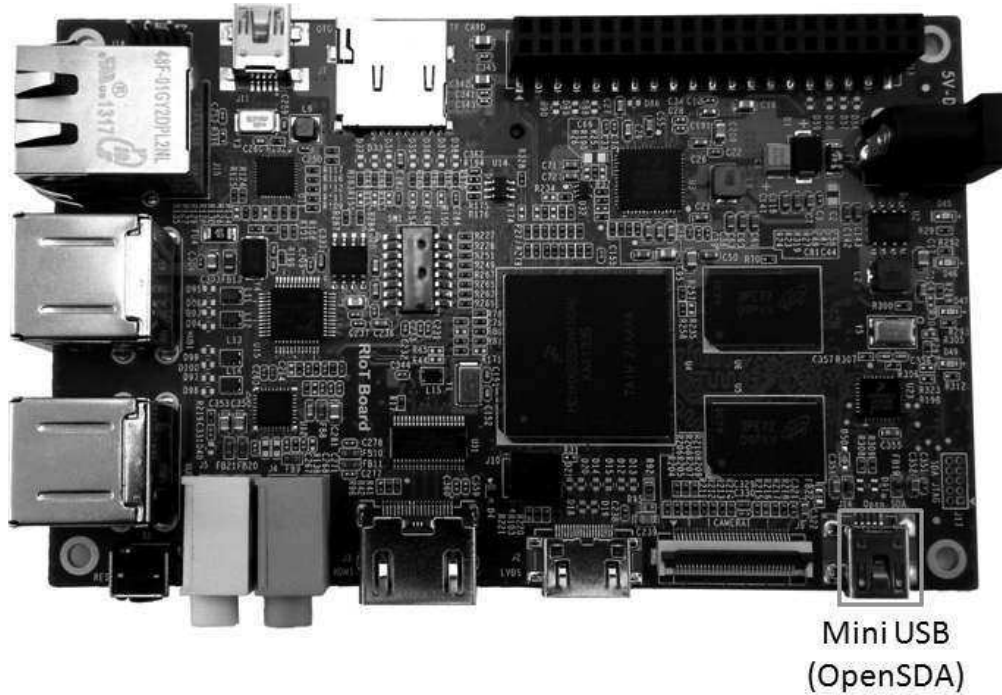
Figure 2-15 Mini USB (OpenSDA)Interface
