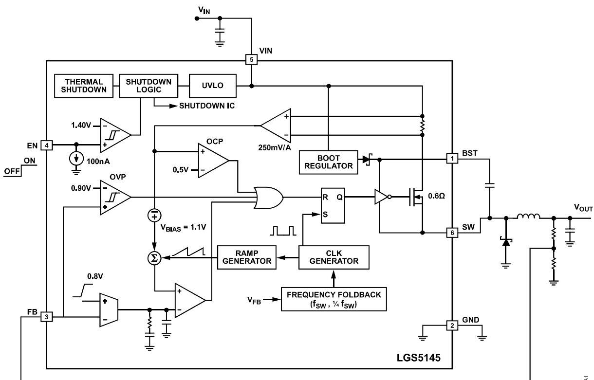
图4 内部框图
