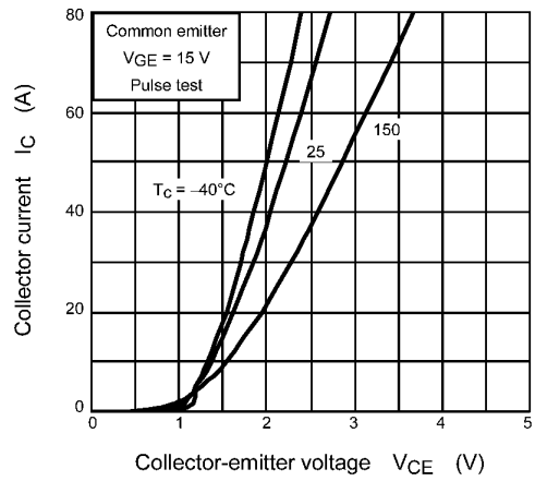
Fig. 8.4 I_C - V_{CE}
