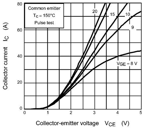
Fig. 8.3 I_C - V_{CE}
