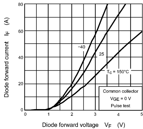
Fig. 8.12 I_F - V_F
