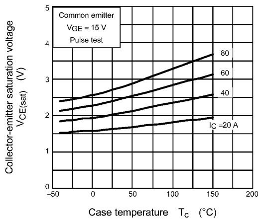
Fig. 8.5 V_{CE(sat)} - T_C
