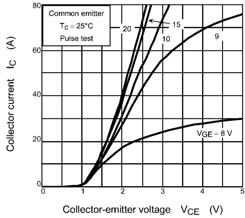
Fig. 8.2 I_C - V_{CE}
