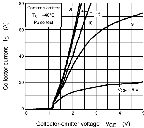
Fig. 8.1 I_C - V_{CE}
