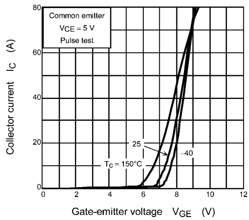
Fig. 8.6 I_C - V_{GE}
