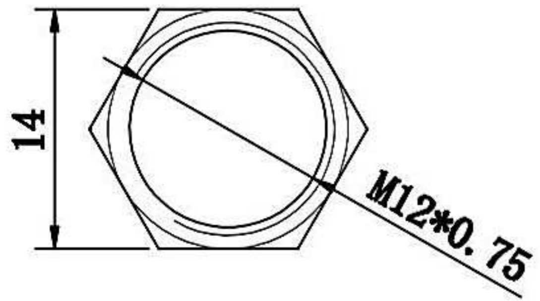
NUT 2 PCS T=2.2
